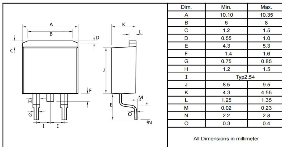
TO-263
